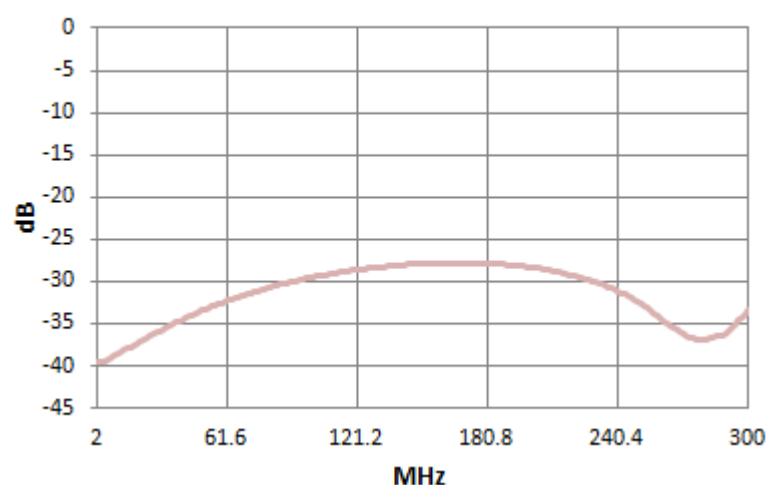
Isolation3-5
